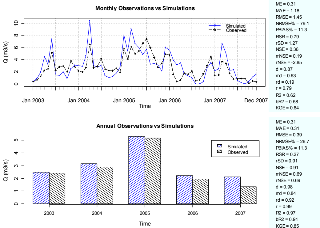
شکل ۵- شبیه‌سازی شده و مشاهداتی ماهانه و سالانه برای ایستگاه سیاه‌آب به همراه شاخص‌های ارزیابی برای دوره اعتبارسنجی.
